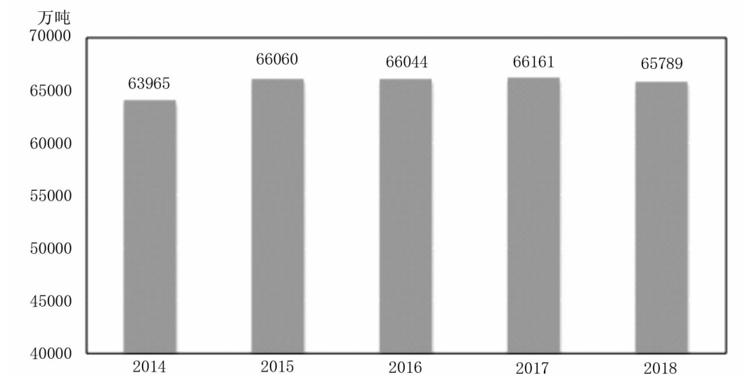
图 9 2014—2018 年粮食产量
